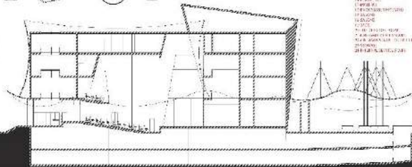
SECTION (A-A) 1:200
